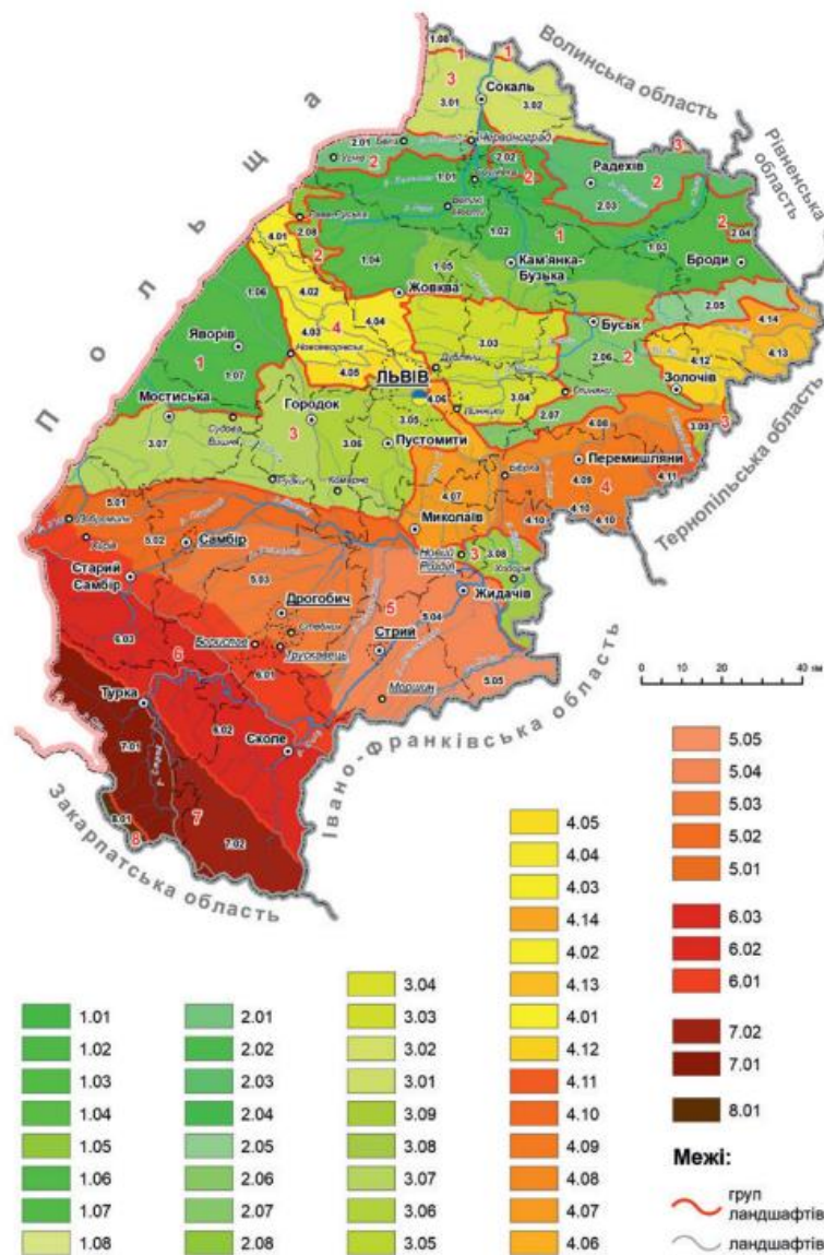
Рис. 2.8. Ландшафтна карта Львівської області
