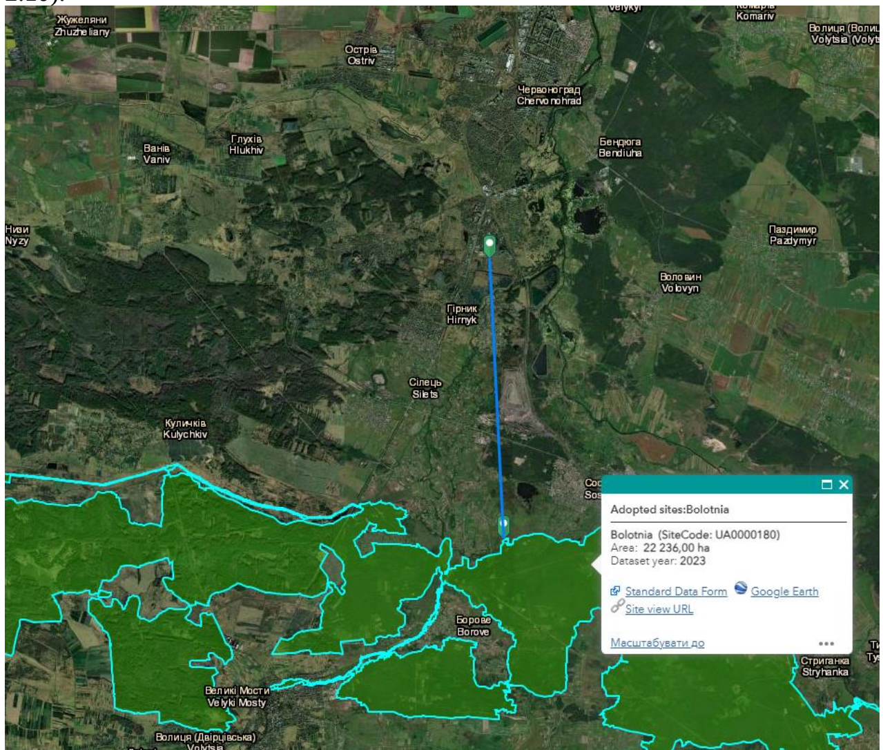
Рис. 2.10. Схематичне розташування проектованої території в системі територій Смарагдової мережі України
