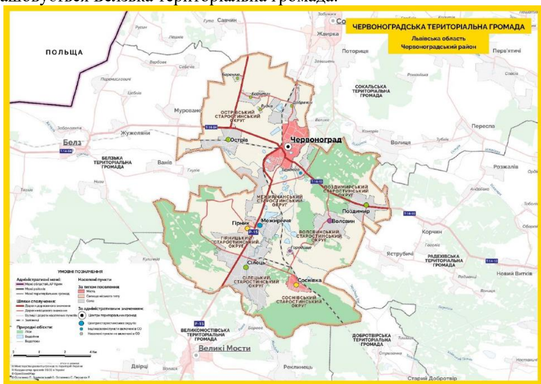
Рис. 2.1. Схема розташування Червоноградської МТГ
