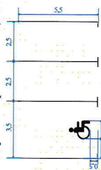
Схема нанесення дорожньої розмітки 1.34, 1.35
