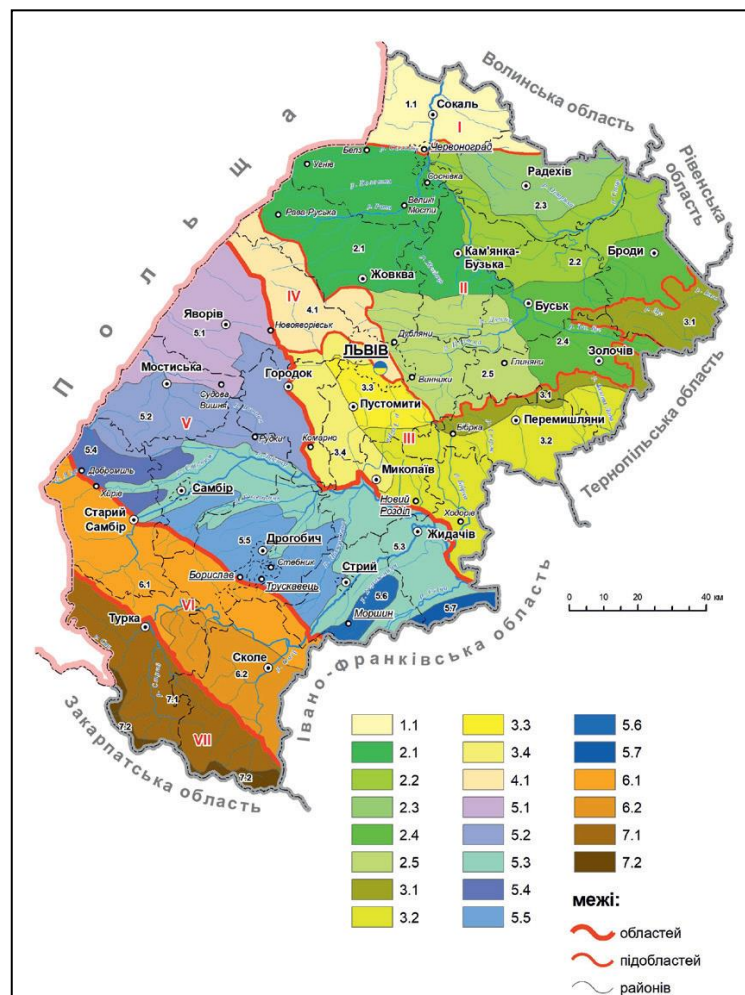
Рис. 2.3. Геоморфологічне районування Львівської області
