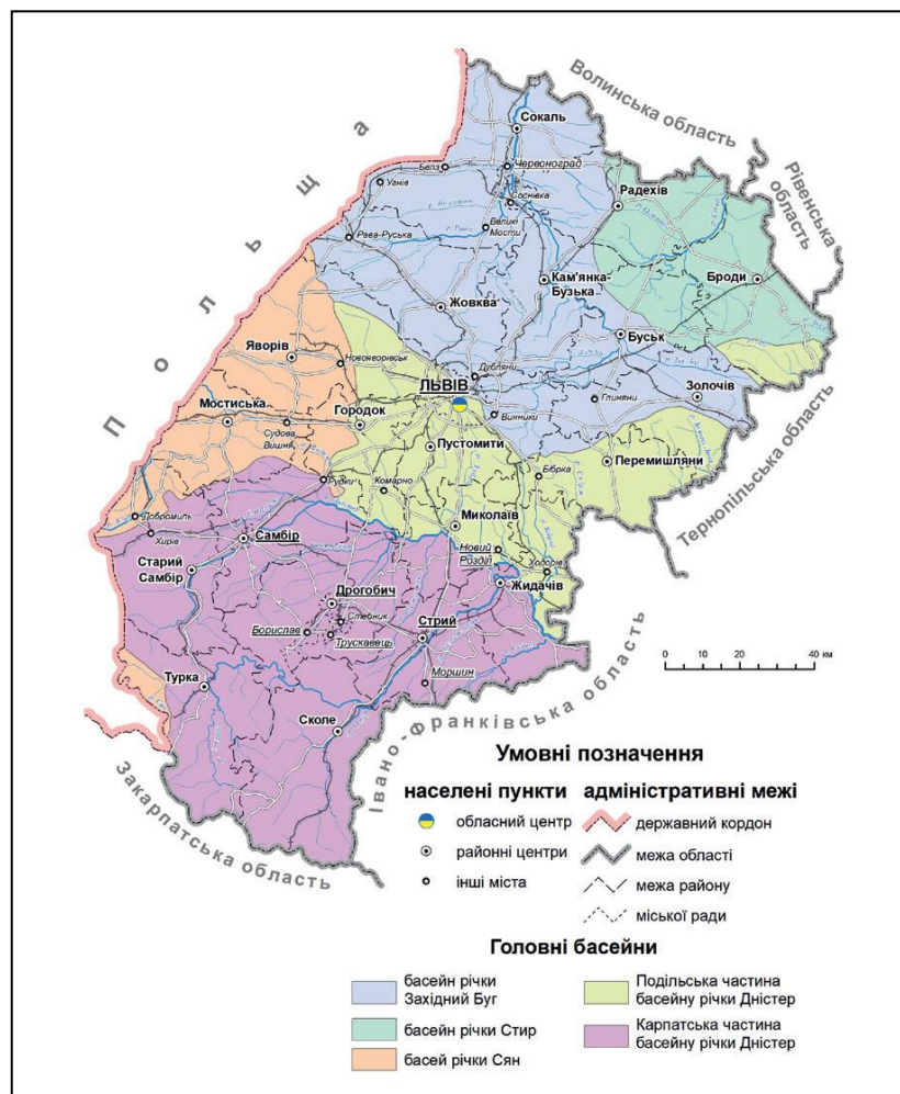
Рис. 2.4. Гідрологічне районування Львівської області
