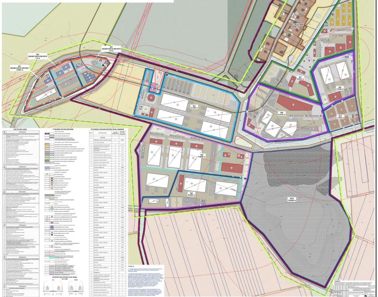
Рис. 4.1. Проектний план території опрацювання ДПТ
